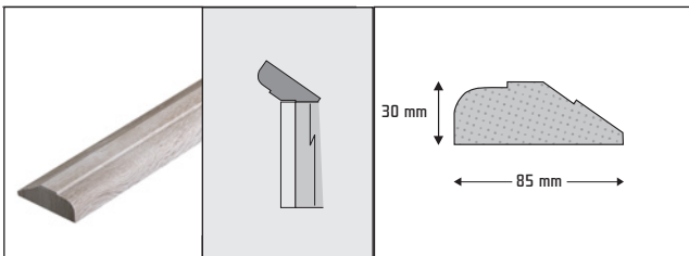
KRANZLEISTE R14 | PLATZIERUNG | PROFIL DER KRANZLEISTE R14
