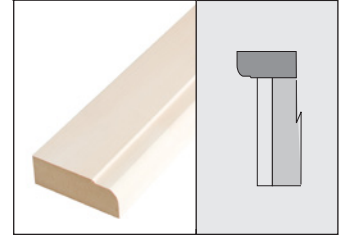
PROFIL DER KRANZLEISTE R4
